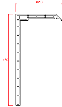
80x160 Pervaz
