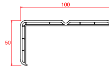
50x100 Pervaz
