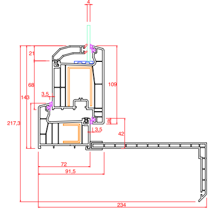
Kasa-Dışa Açılım Kapı
