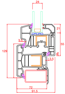
Orta Kayıt-Damlalıkli Kanat
