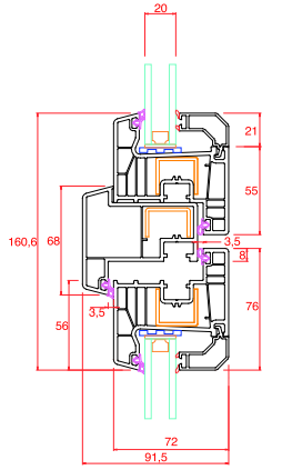
Hareketli Orta Kayıt-Kanat
