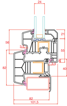
Orta Kayıt-Damlalıklı Kanat
