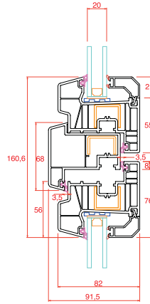
Hareketli Orta Kayıt-Kanat
