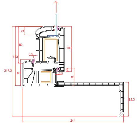
Kasa-Dışa Açılım Kapı
