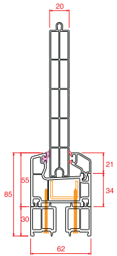
Yükseltme-Kasa
