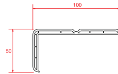
50x100 Pervaz
